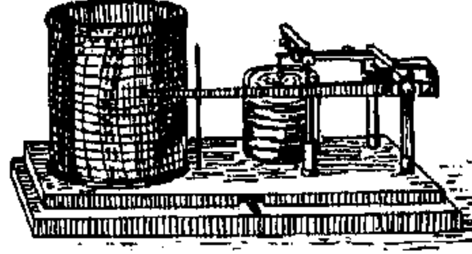
مرسمة الضّغط
